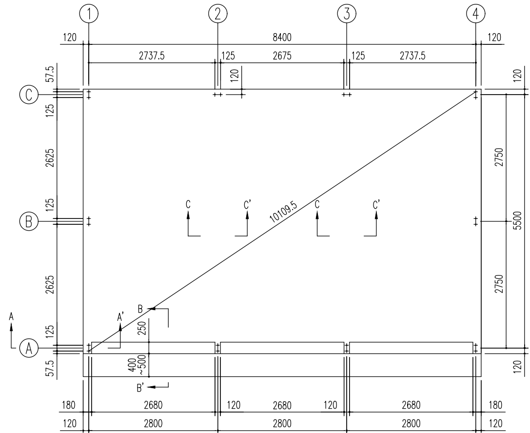
基礎伏図(S= 1/80)
