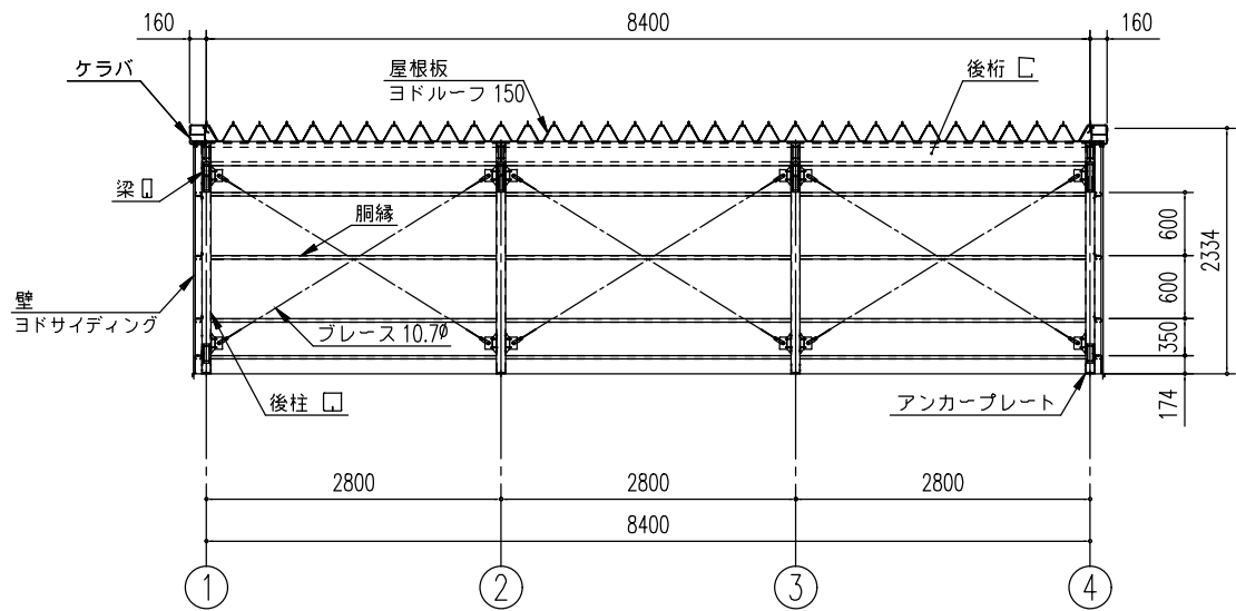
正面断面図 (S= 1/80)
