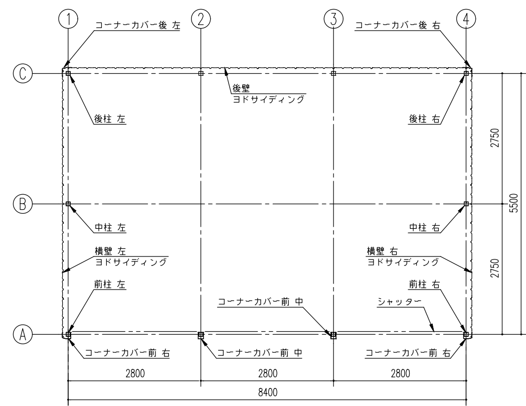
平面図 (S= 1/80)
