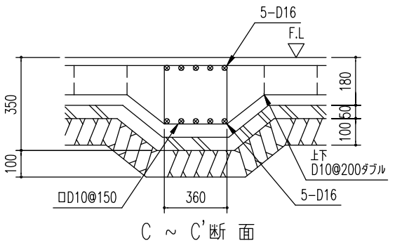
ベタ基礎断面図 (S = 1/20)
