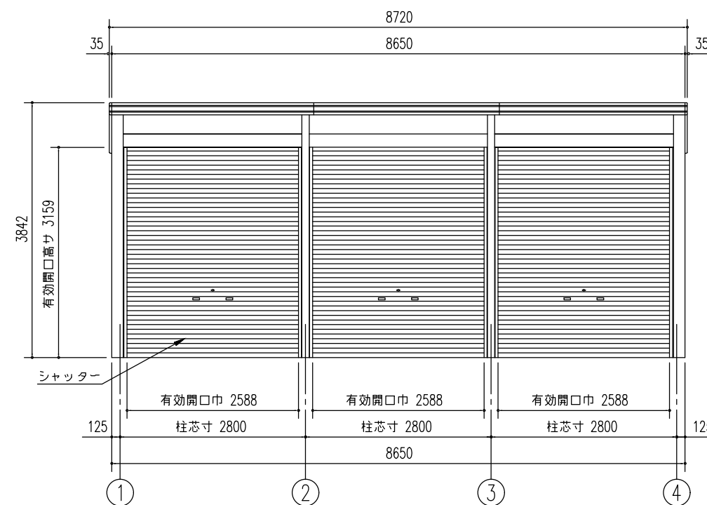
正面立面図 (S=1/80)
