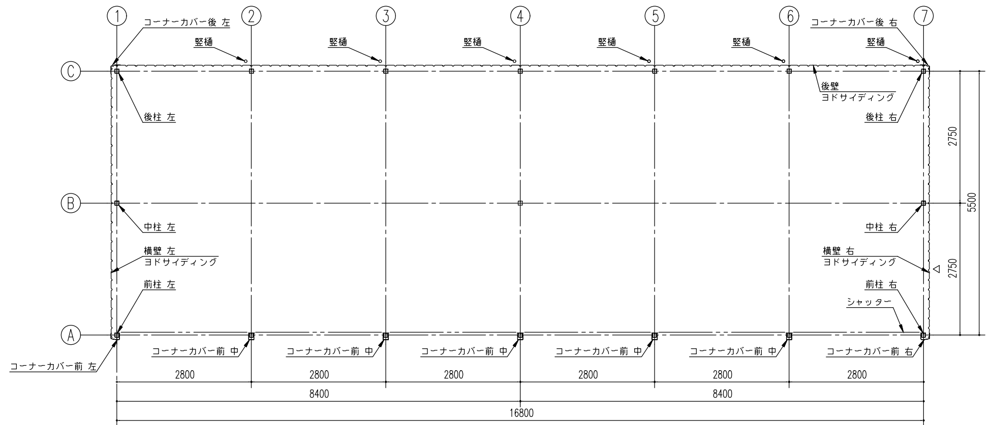
平面図 (S=1/80)
