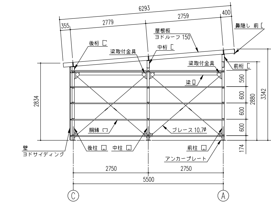
側面断面図 (S= 1/80)
