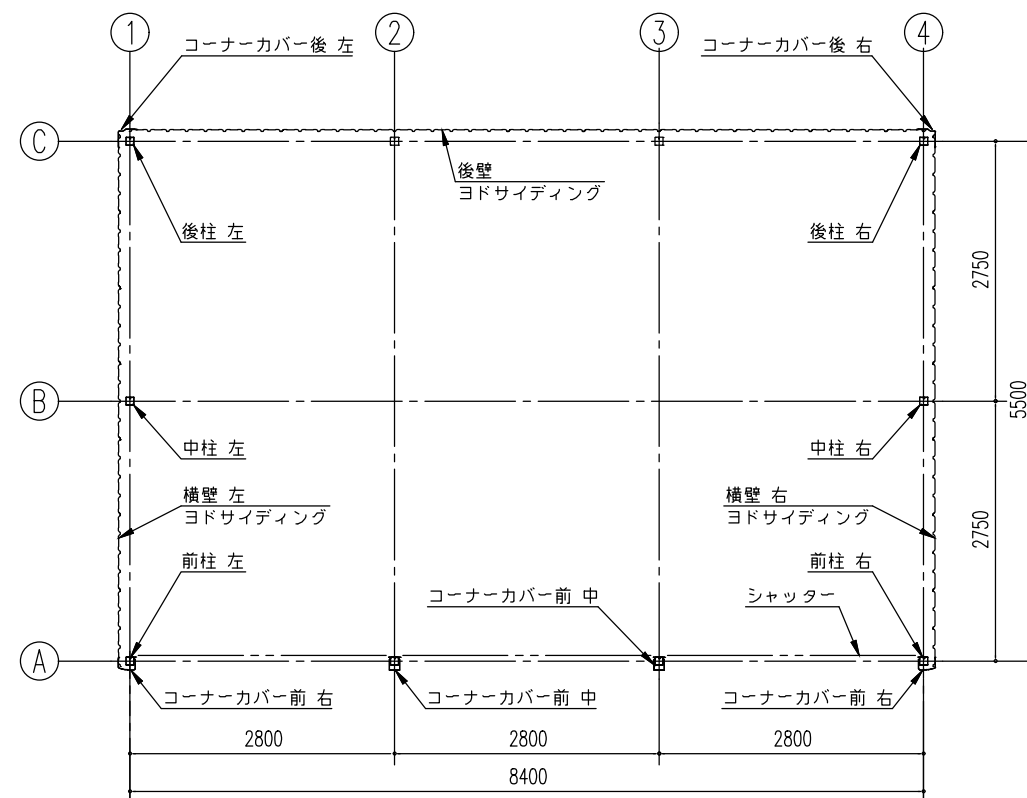
平面図 (S=1/80)
