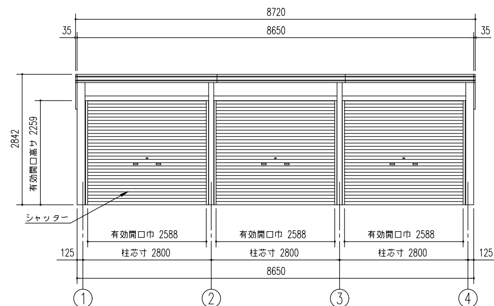
正面立面図(S= 1/80)
