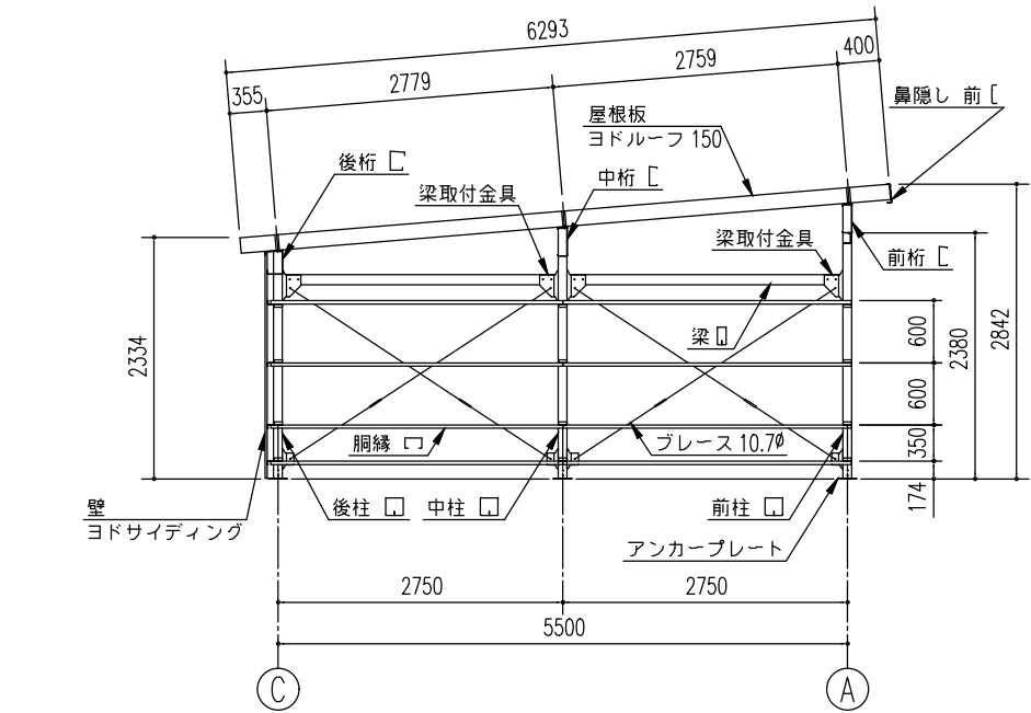
側面断面図 (S= 1/80)
