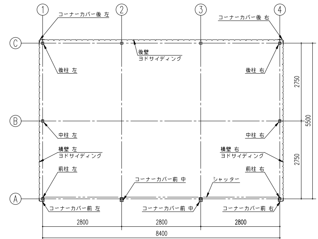
平面図 (S=1/80)
