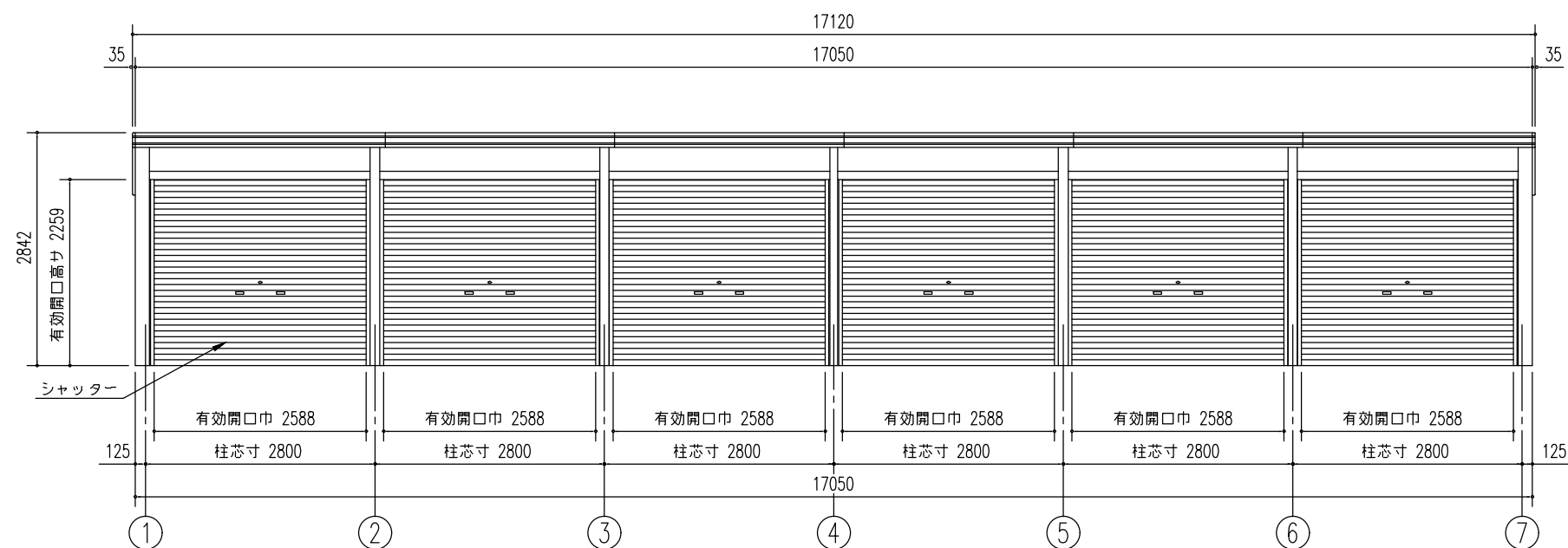
正面立面図(S= 1/80)
