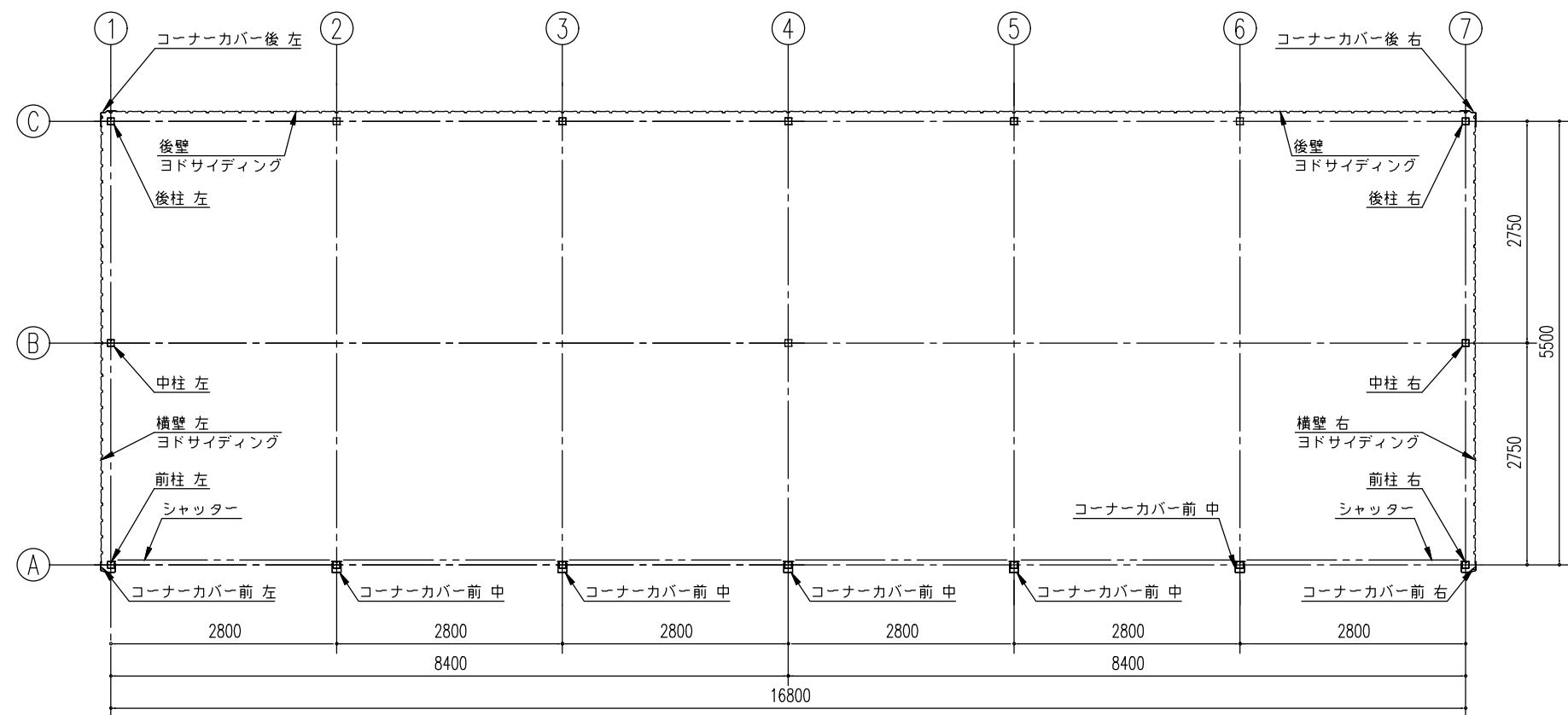
平面図 (S= 1/80)
