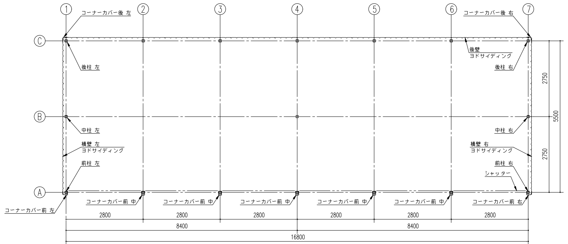
平面図 (S= 1/80)
