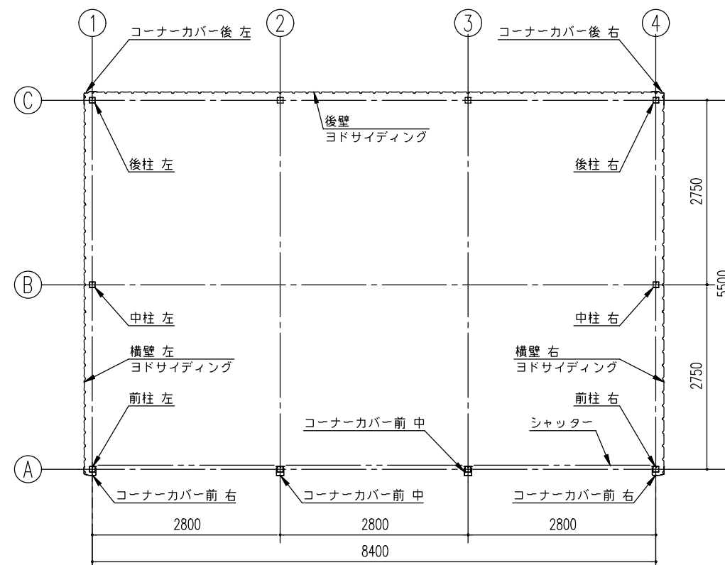
平面図 (S= 1/80)
