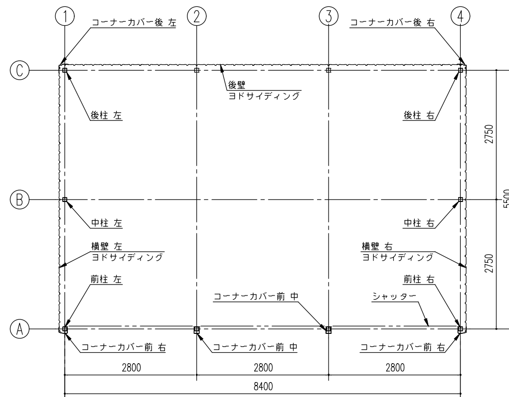
平面図 (S=1/80)
