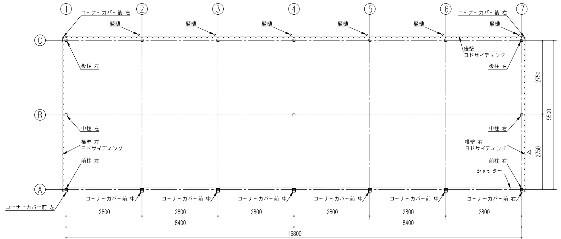
平面図 (S= 1/80)
