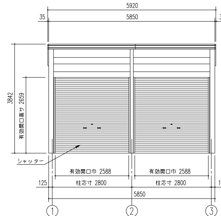
正面立面図 (S=1/80)
