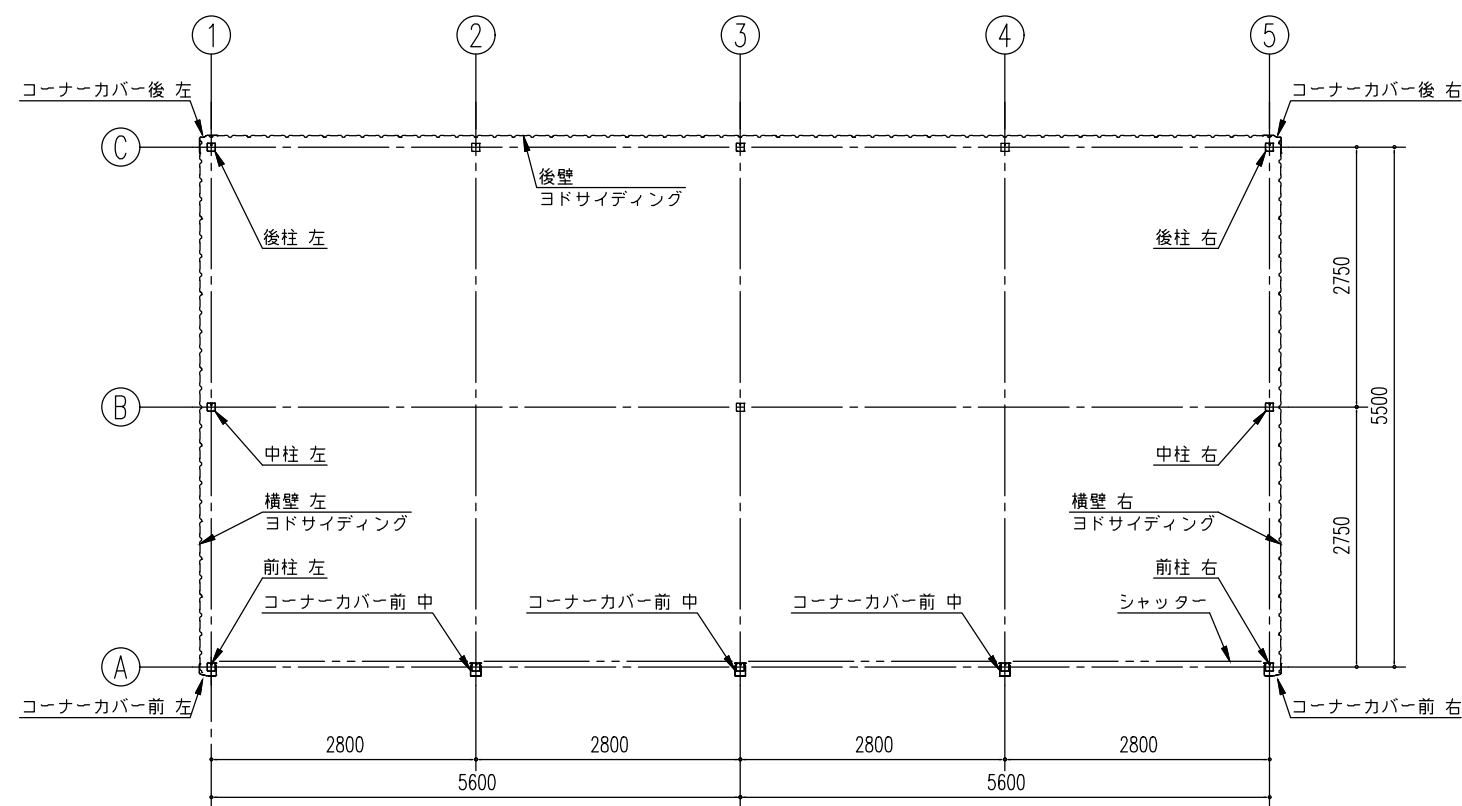
平面図 (S=1/80)
