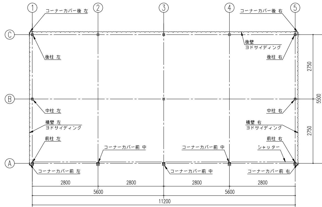
平面図 (S=1/80)
