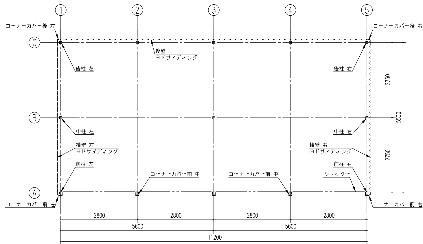
平面図 (S=1/80)
