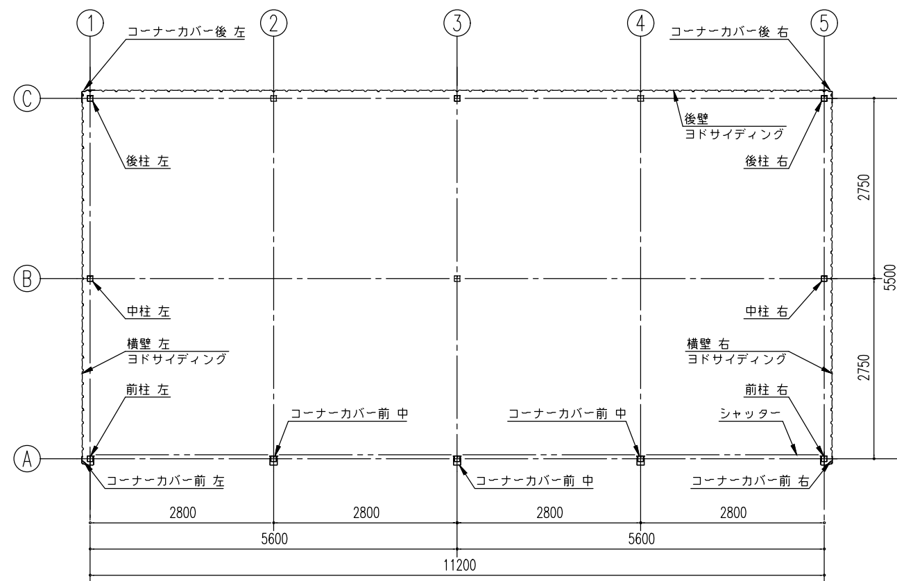
平面図 (S=1/80)
