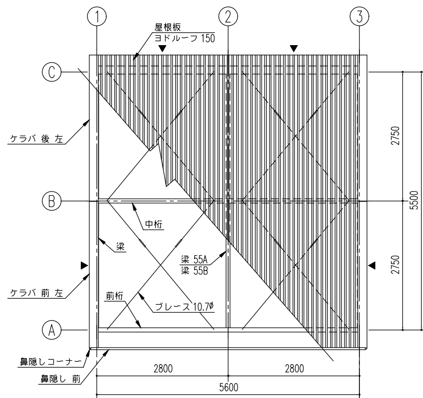
小屋伏図 (S=1/80) ▶は、プレース 10.7φ とする。
