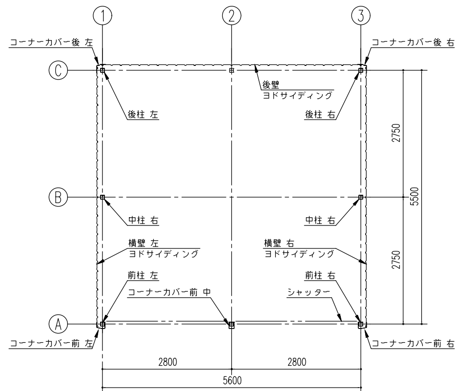
平面図 (S=1/80)
