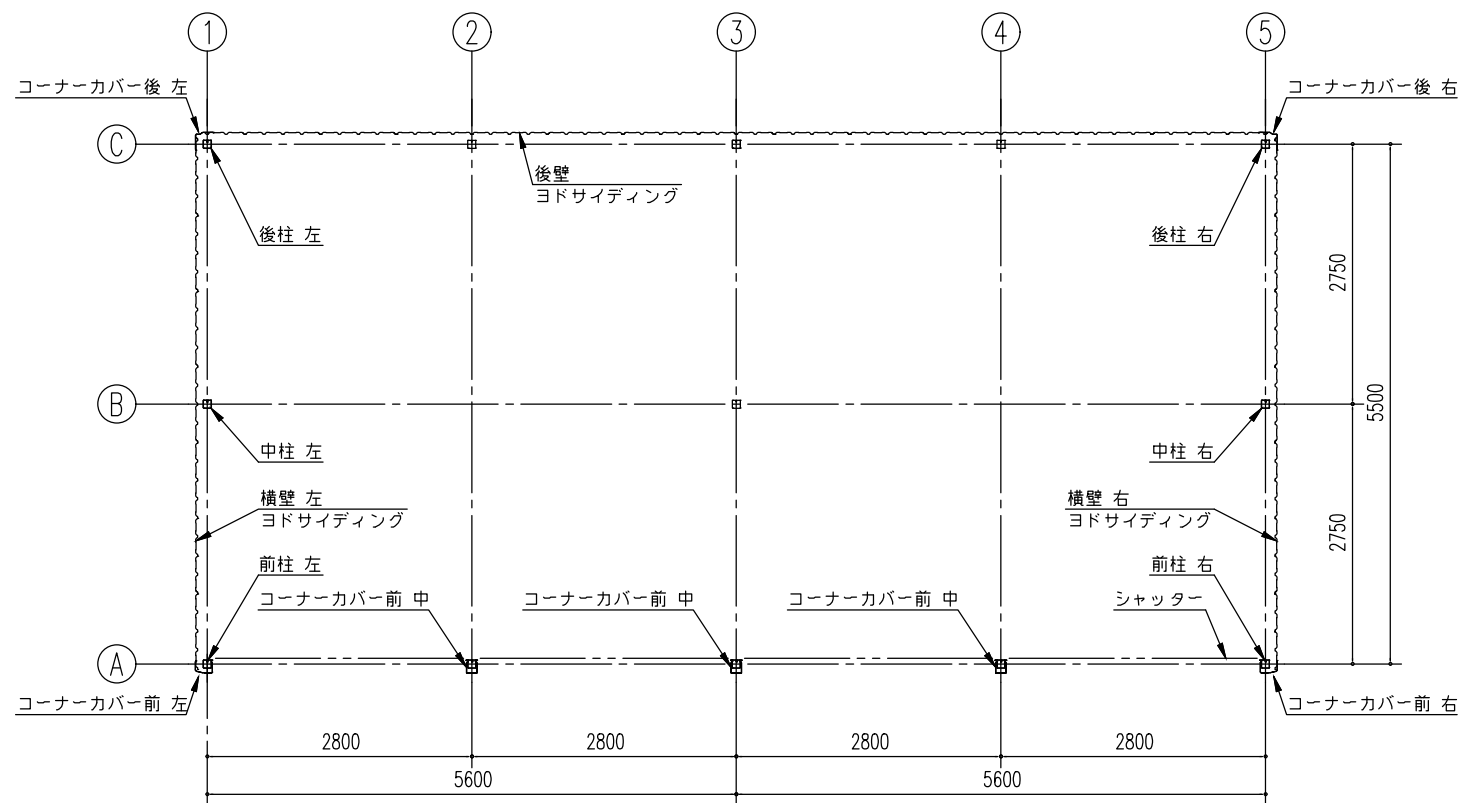
平面図 (S=1/80)
