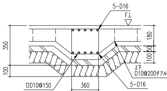
C ~ C' 断面
