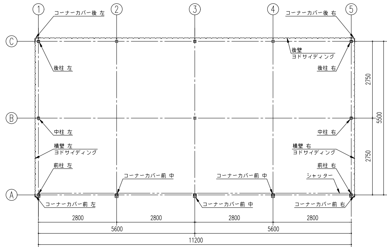
平面図 (S=1/80)
