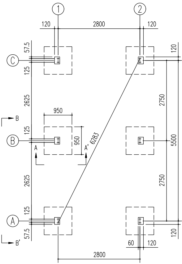
基礎伏図 (S=1/80)
