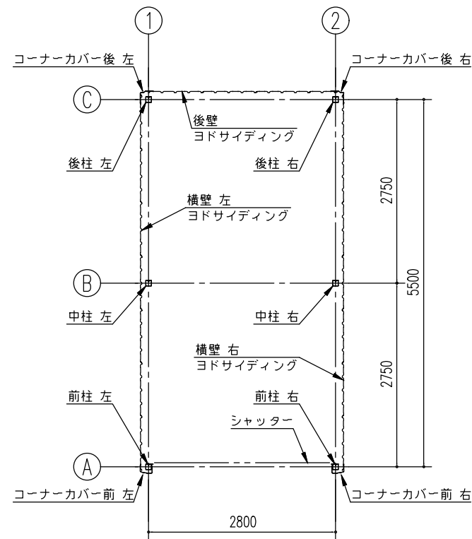
平面図 (S= 1/80)
