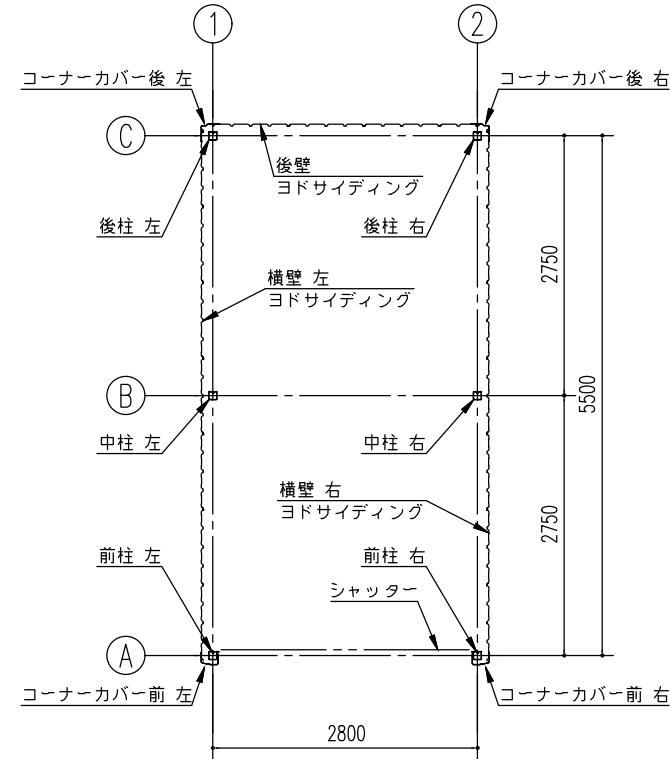
平面図 (S=1/80)
