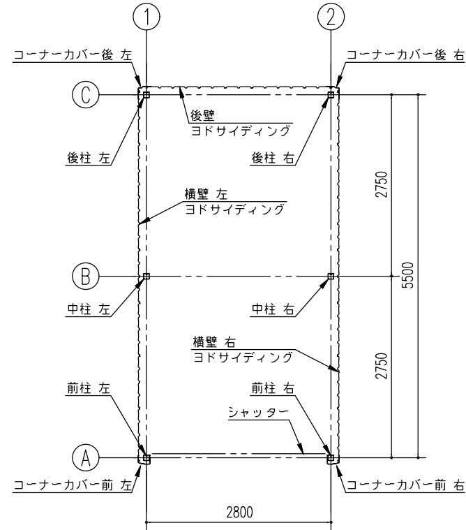
平面図 (S=1/80)
