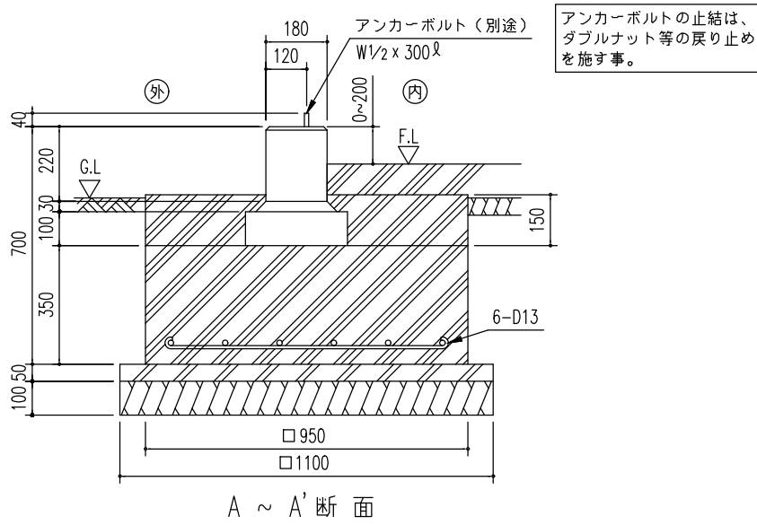
独立基礎断面図 (S = 1/20)
