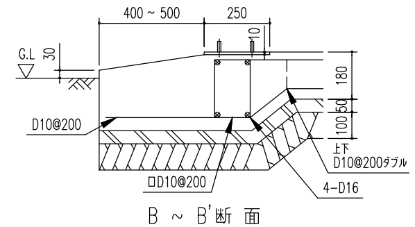
ベタ基礎断面図 (S = 1/20)
