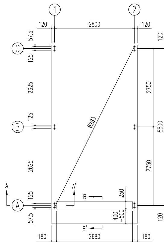
基礎伏図 (S=1/80)
