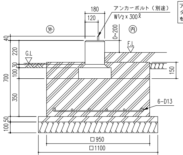
A ~ A' 断面
