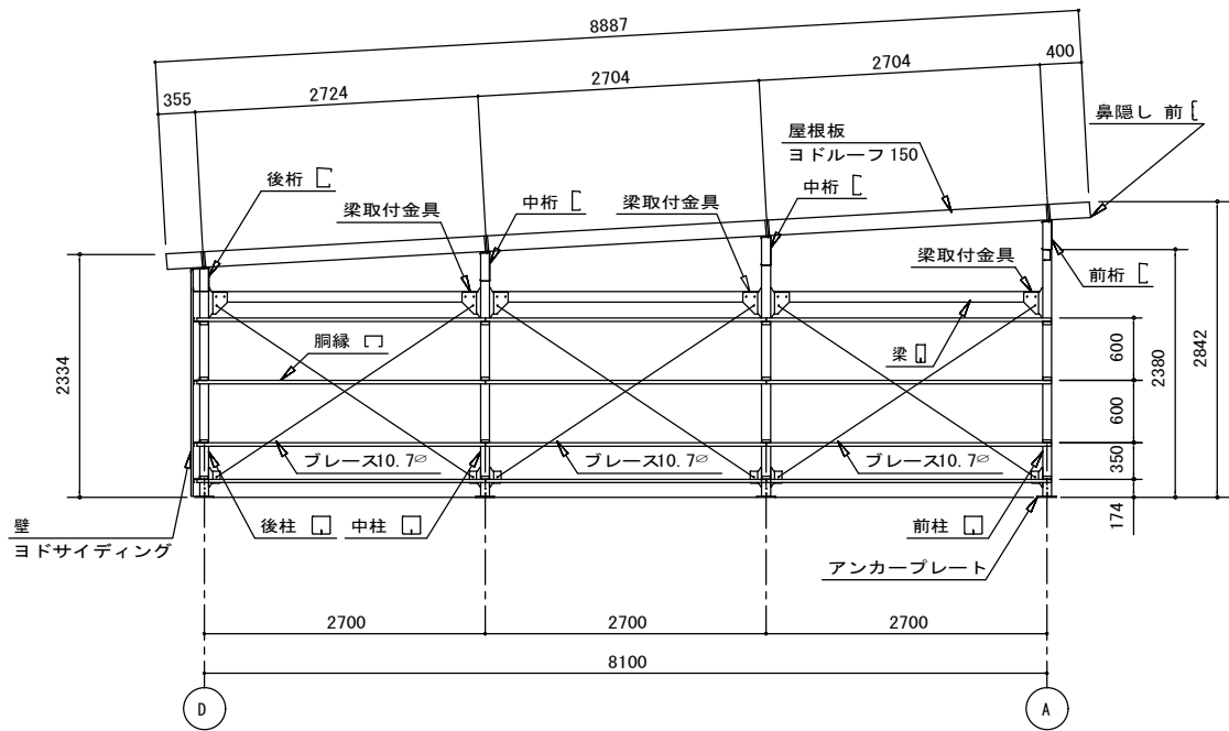
側面断面図 S=1/80
