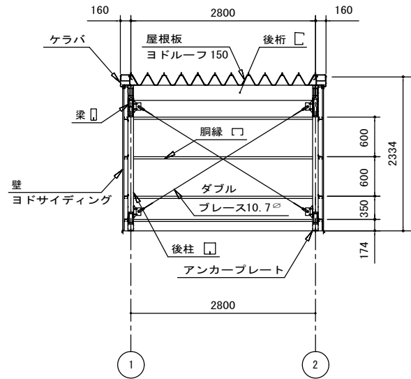
正面断面図 S=1/80
