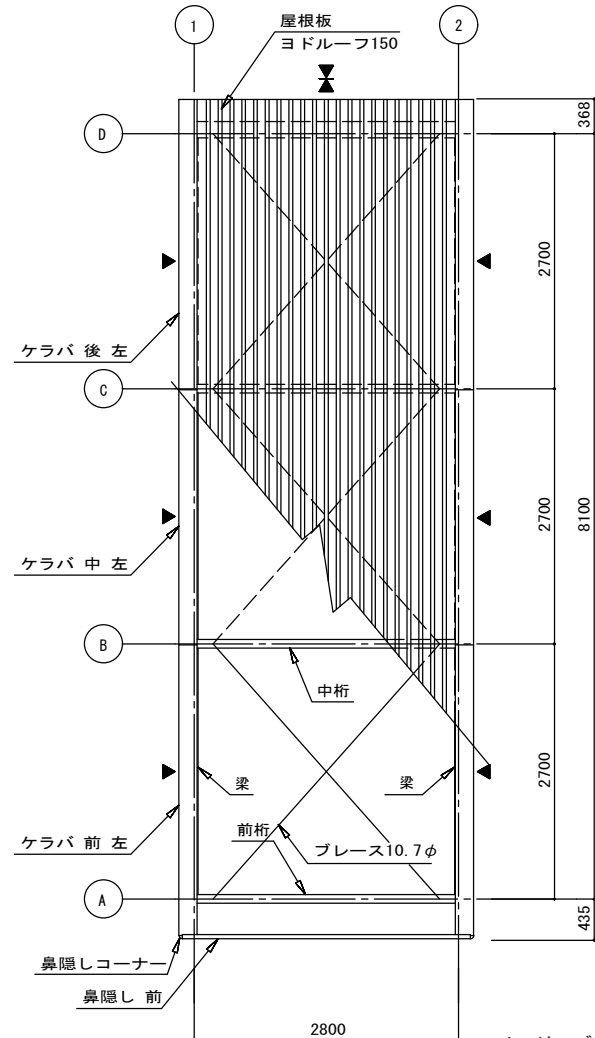
小屋伏図 S=1/80
