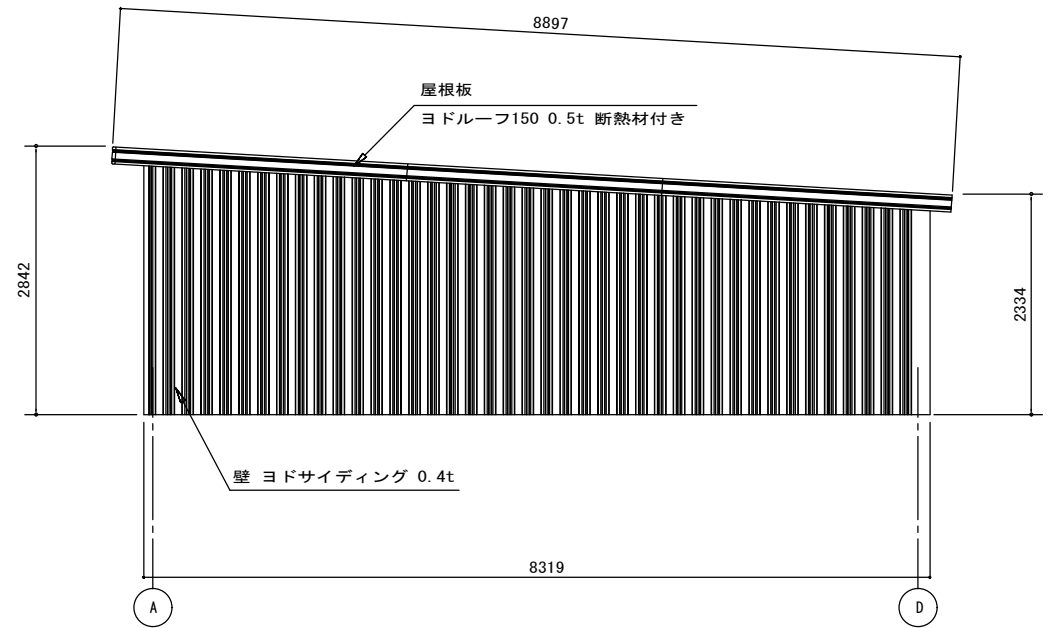
側面立面図 S=1/80
