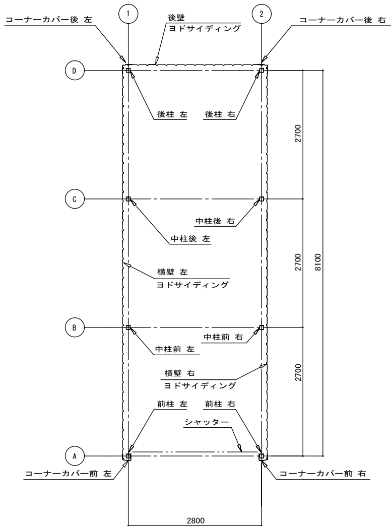
平面図 S=1/80
