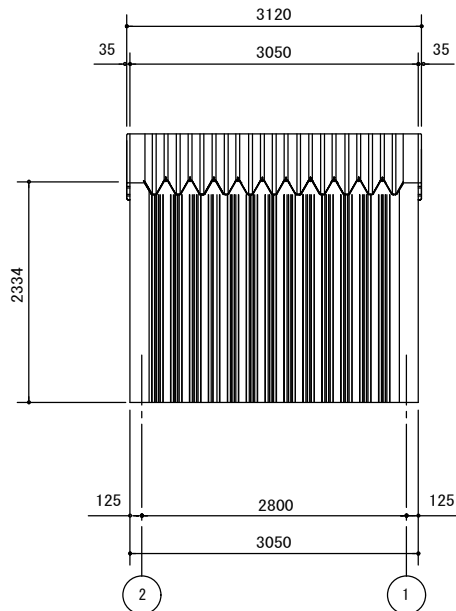
後面立面図 S=1/80
