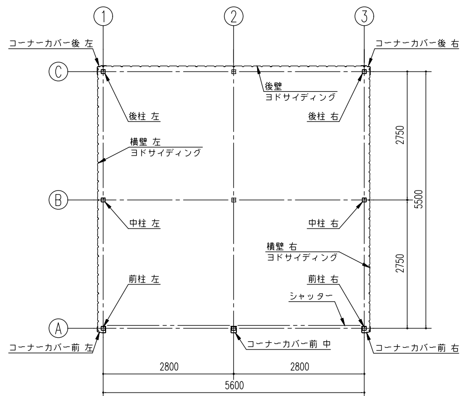
平面図 (S=1/80)
