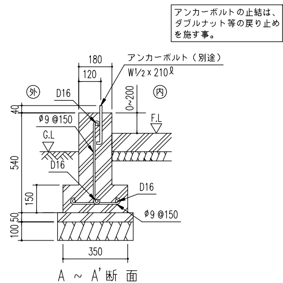
布基礎断面図 ( S = 1/20 )
