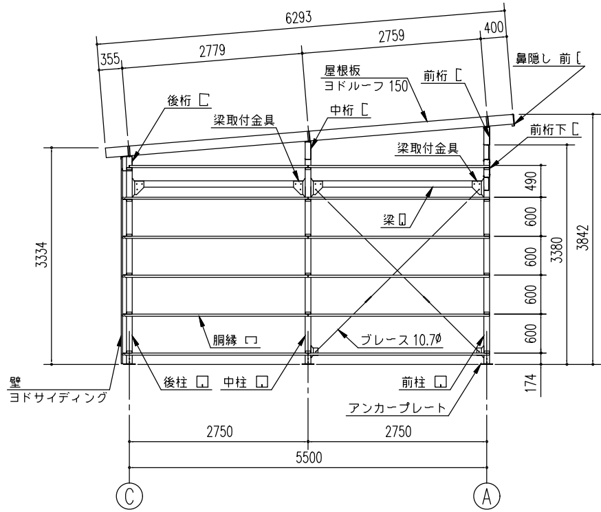
側面断面図 (S= 1/80) ※側面の出入口により、ブレースの配置が 変更となる場合があります。
