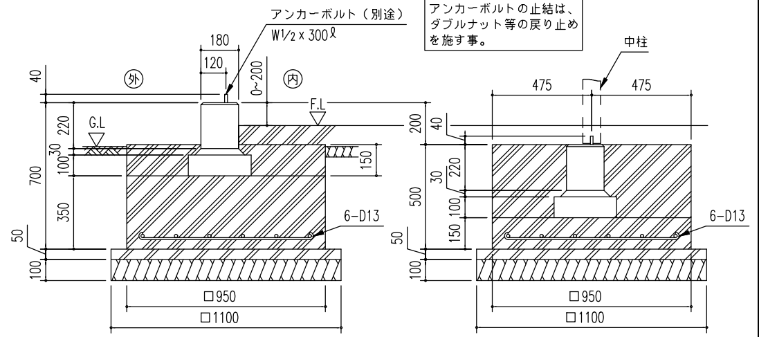
A ~ A'断面
