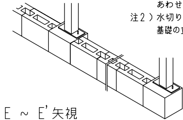
E ~ E' 矢視
