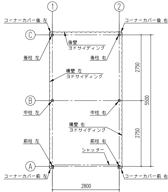
平面図 (S=1/80)
