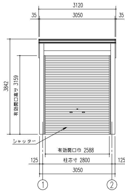
正面立面図 (S=1/80)
