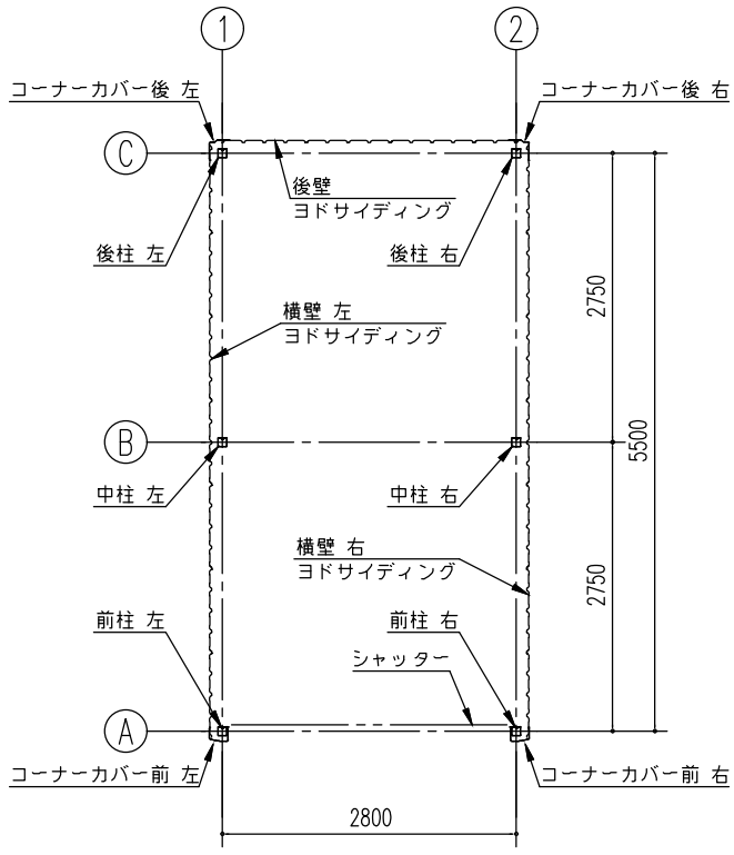
平面図 (S=1/80)
