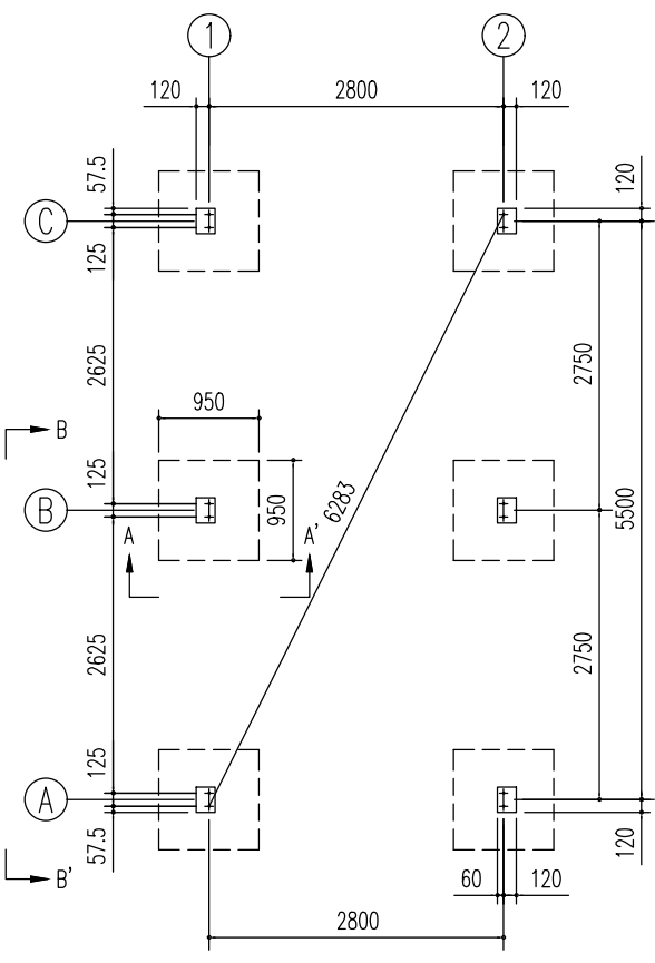
基礎伏図 (S= 1/80)
