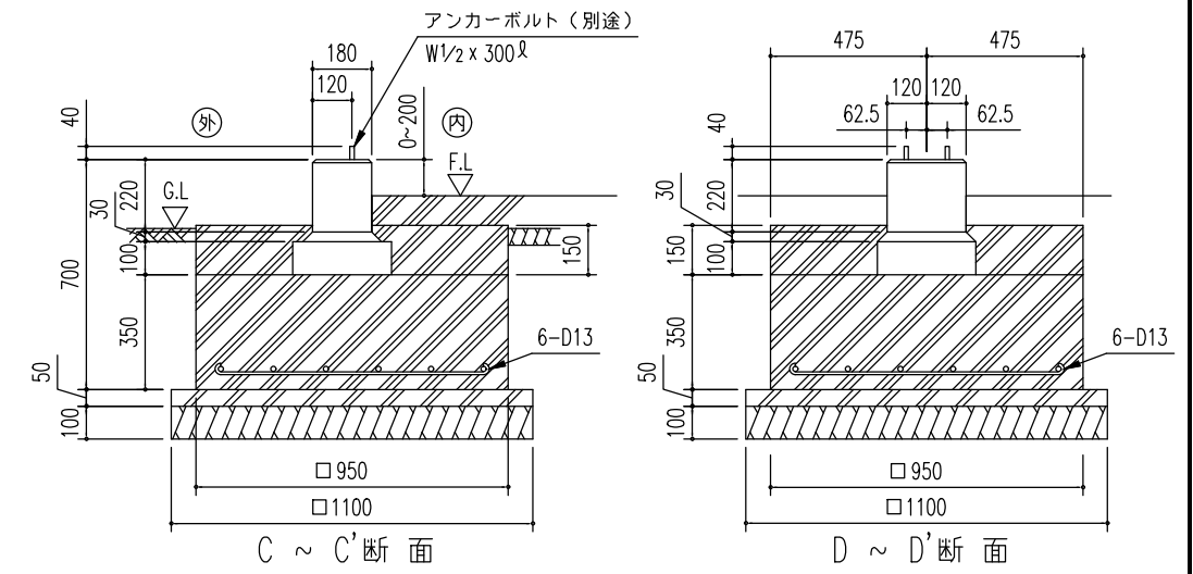
独立基礎断面図 (S = 1/25) <下記条件での参考図> (地耐力 50 kN/m 2 以上,コンクリート設計基準強度 18 N/mm 2 以上) (基準風速 34 m/s, 地表面粗度区分 Ⅲ)
