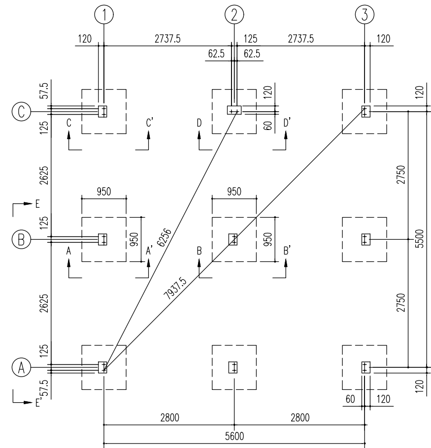
基礎伏図 (S= 1/80)
