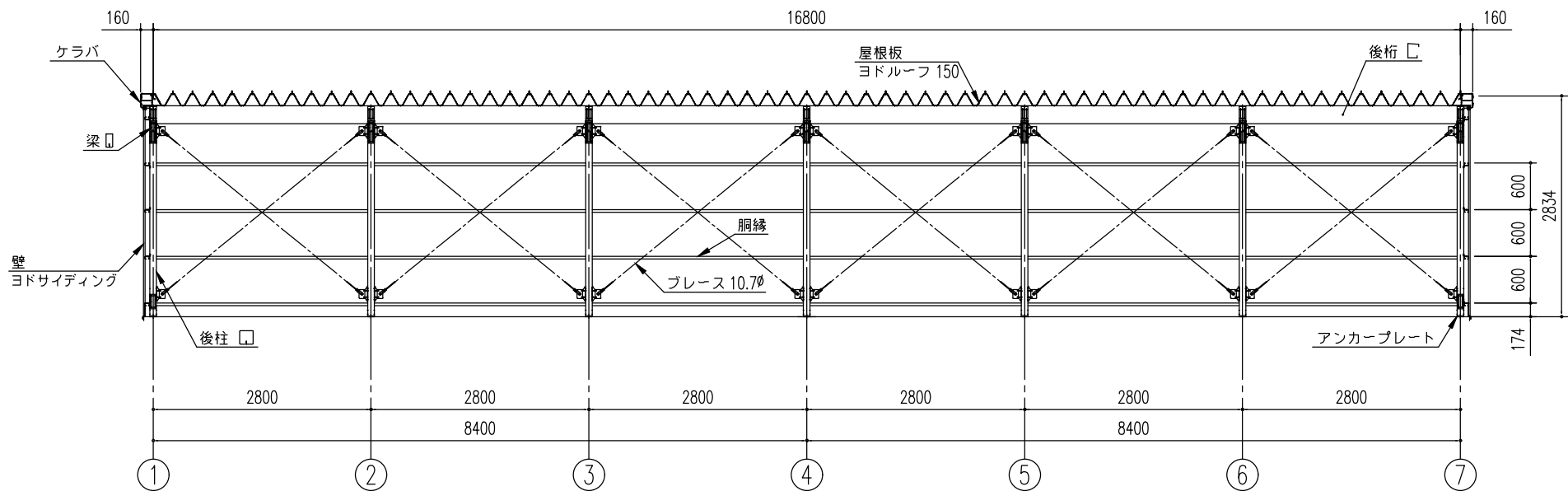
正面断面図 (S=1/80)
