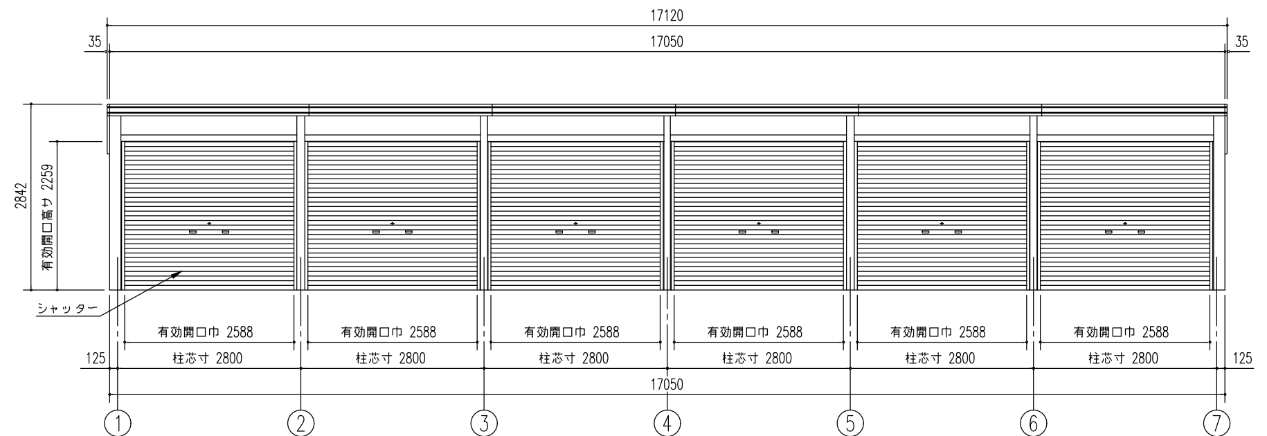
正面立面図 (S= 1/80)
