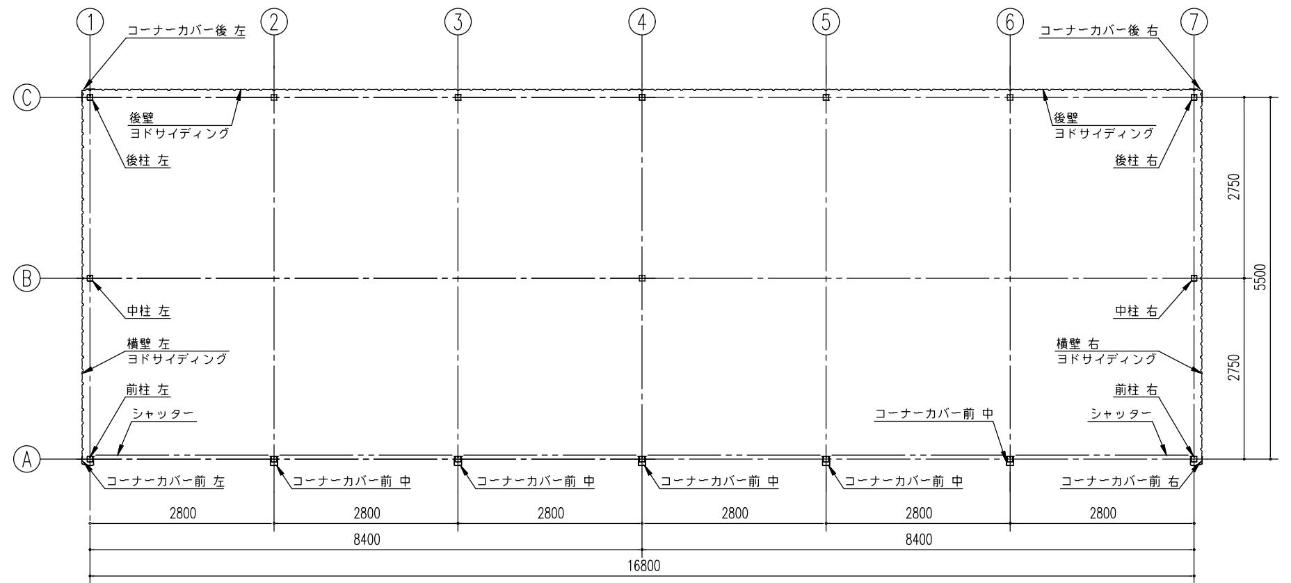
平面図 (S= 1/80)
