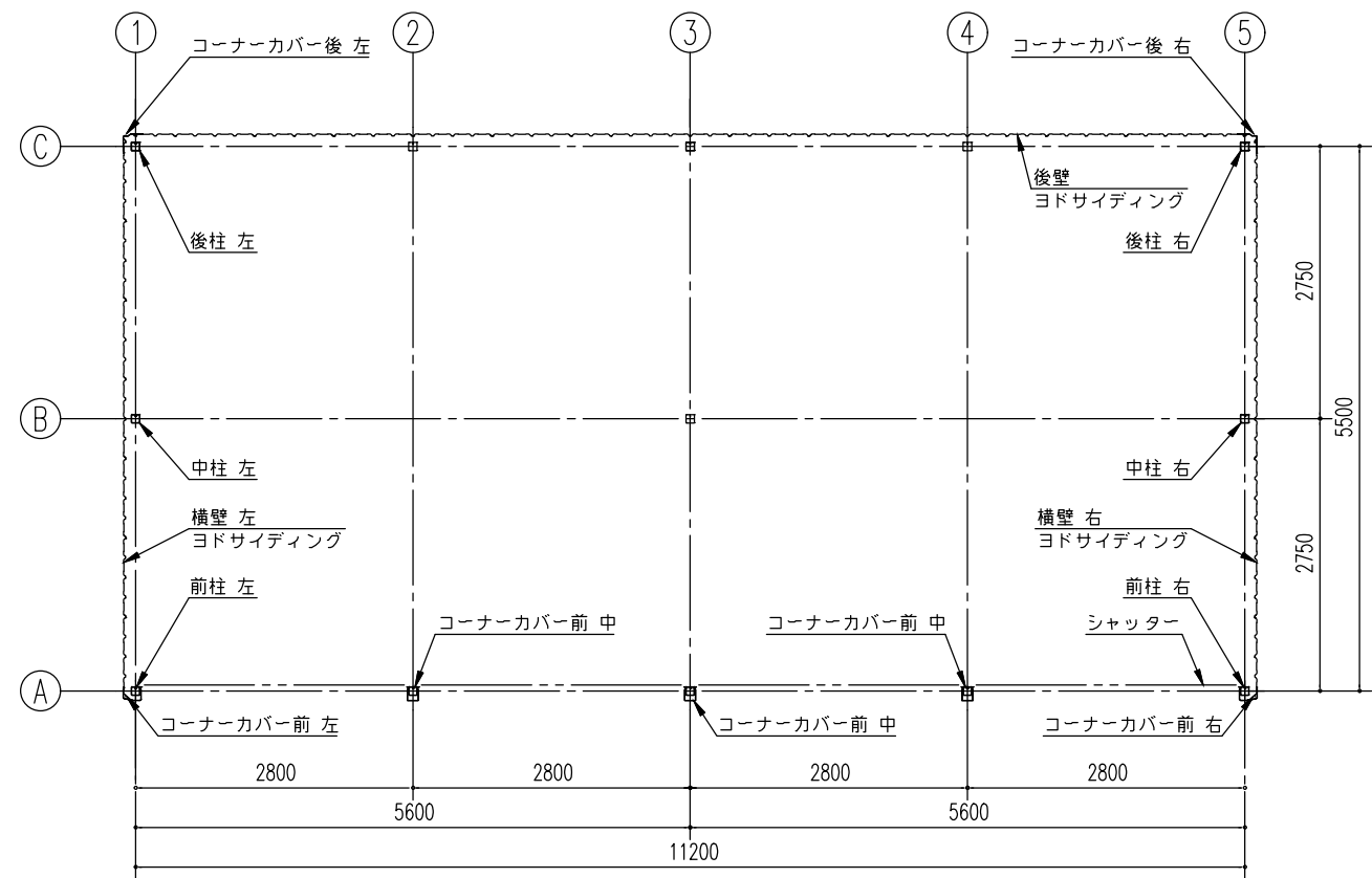
平面図 (S=1/80)
