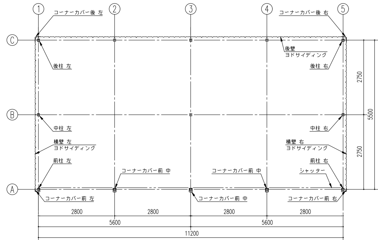
平面図 (S=1/80)
