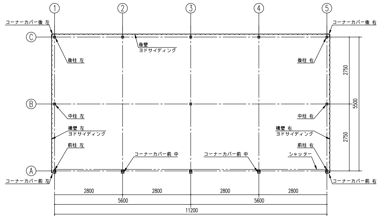
平面図 (S=1/80)
