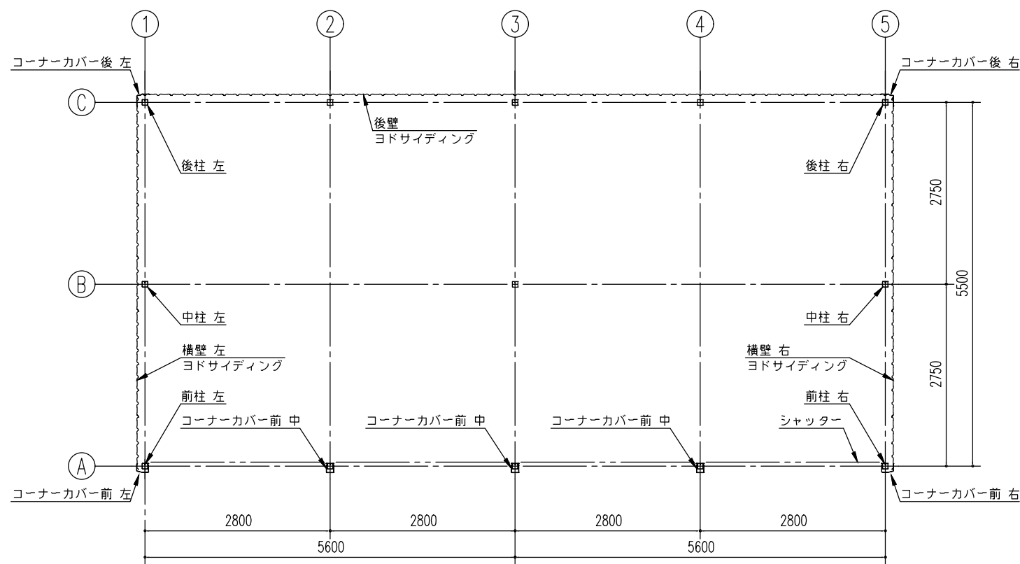
平面図 (S= 1/80)
