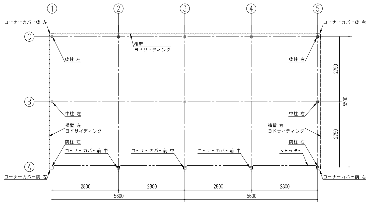
平面図 (S= 1/80)
